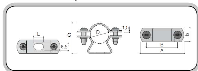
disegno dimensionale / reference details
